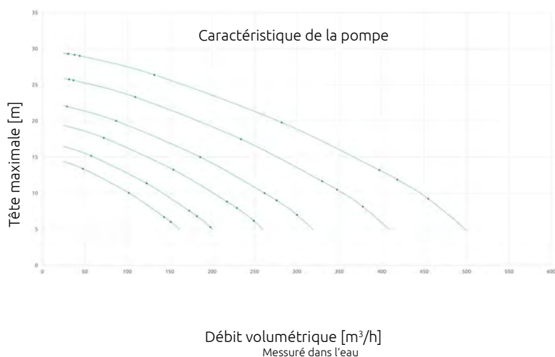
Réglage du pompage
