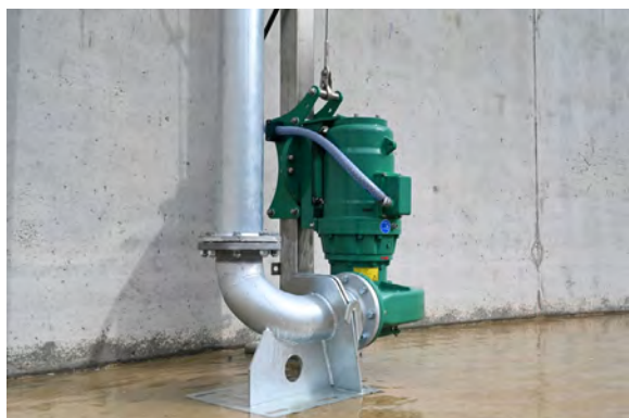
PRESSURA TP - Cuve en béton
