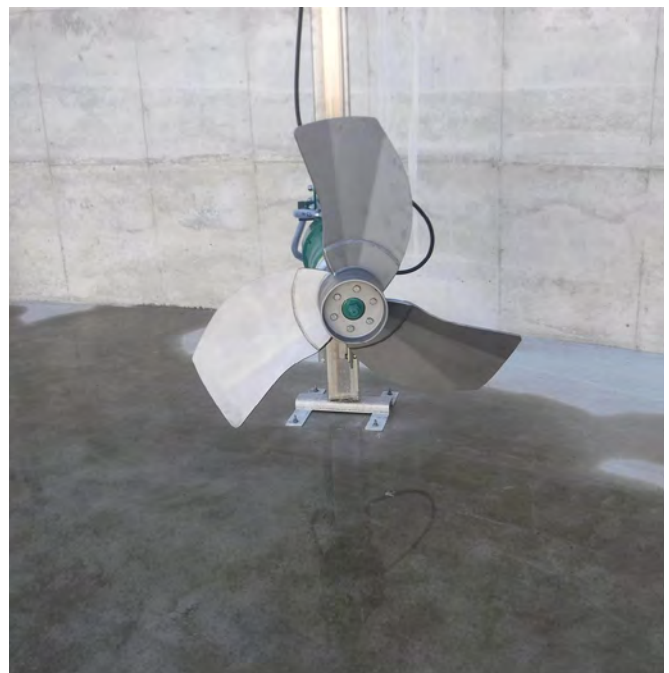
4G avec EV - Cuve ouverte
